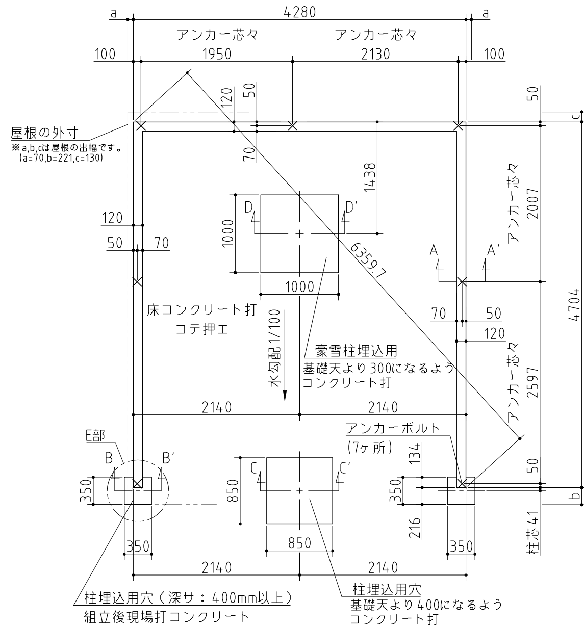
基礎詳細図 S=1/20
